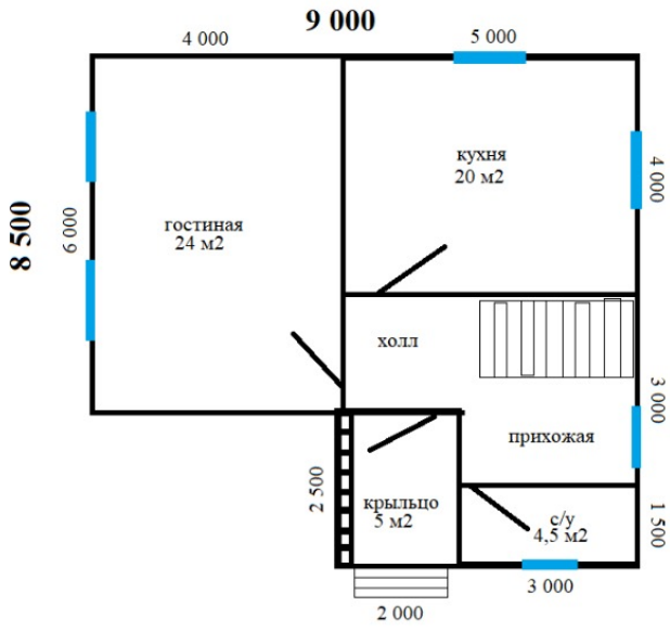
План 1 этажа
