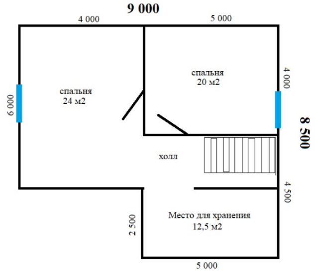
План 2 этажа
