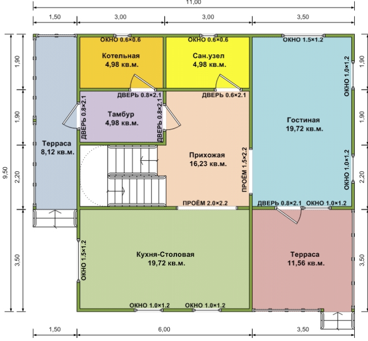
План 1-ого этажа
